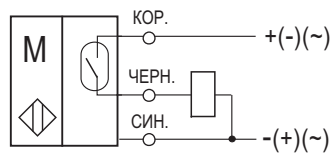
Схема подключения нагрузки
