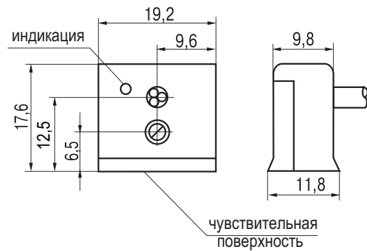
Габаритный чертёж
